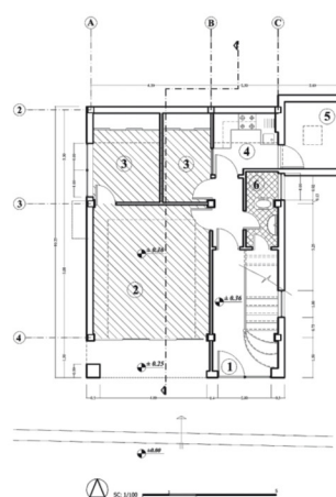
نقشه طبقه همکف Ground floor plan
