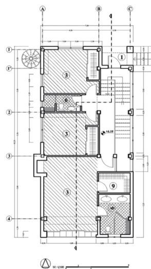
نقشه طبقه دوم Second floor plan
