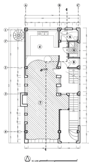
نقشه طبقه اول First floor plan
